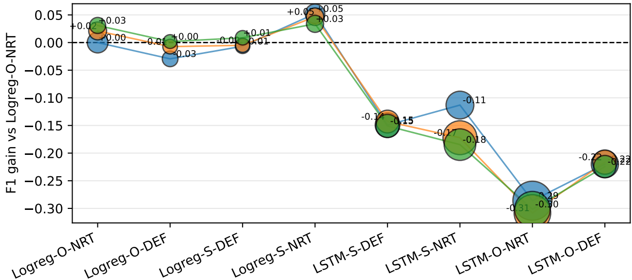
F1 gain, 2022-01-01 to 2025-01-01
