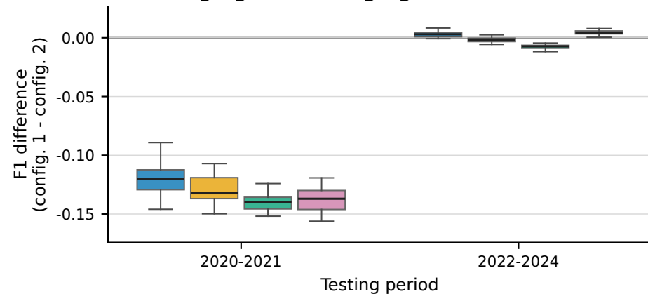
b F1: Logreg-S-DEF - Logreg-O-DEF
