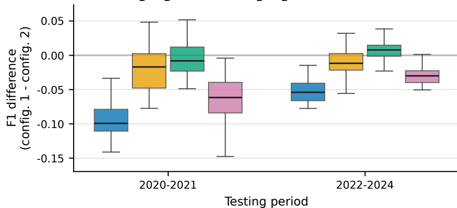
b F1: Logreg-S-NRT - Logreg-O-NRT
