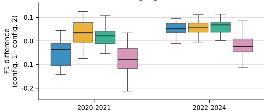
b F1: LSTM-O-NRT - Logreg-O-NRT
