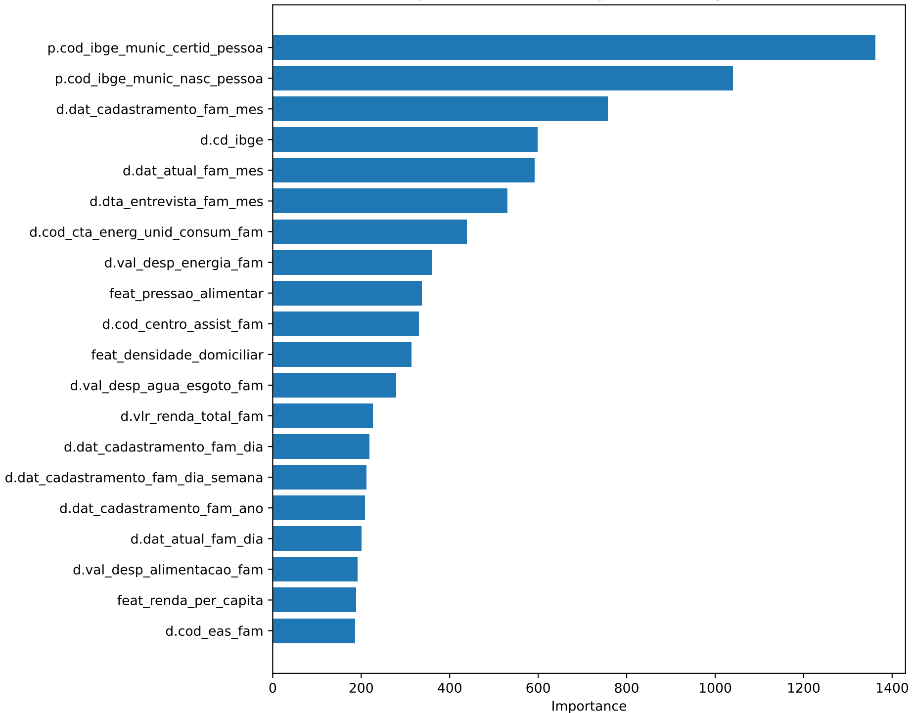
Top 20 variáveis mais importantes — LightGBM
