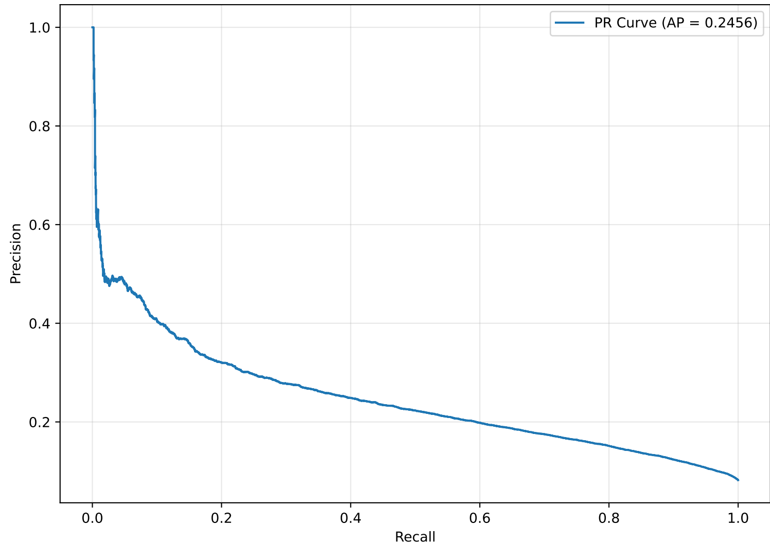
Curva Precision-Recall — Baseline de validação (LightGBM)
