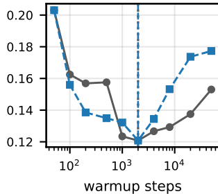
ETTm2 / PatchTST
