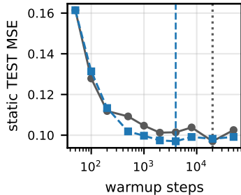
ETTm2 / DLinear
