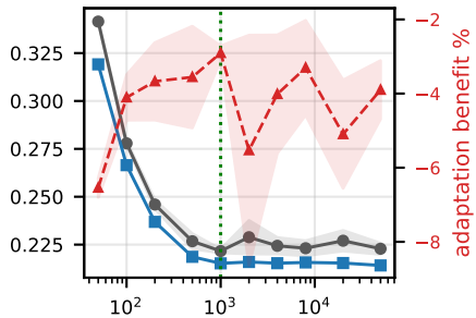
BDG2 / PatchTST
