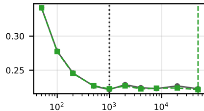
BDG2 / PatchTST
