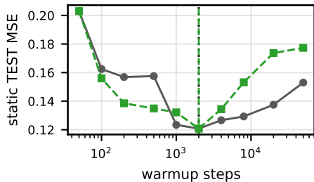
ETTm2 / PatchTST
