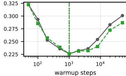
BDG2 / PatchTST
