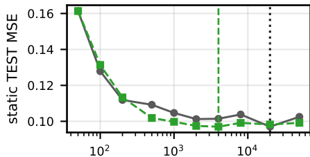
ETTm2 / PatchTST
