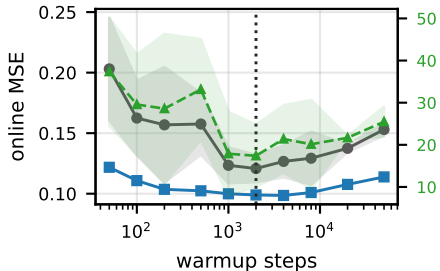
ETTm2 / PatchTST
