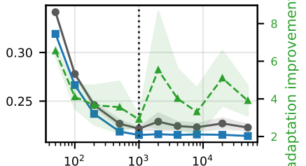
BDG2 / DLinear
