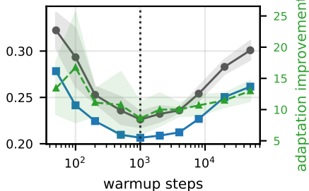
BDG2 / PatchTST
