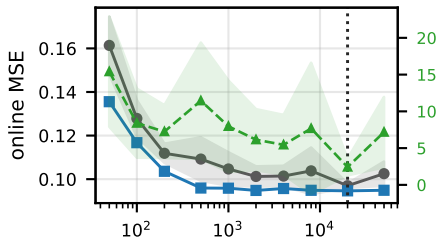
ETTm2 / DLinear
