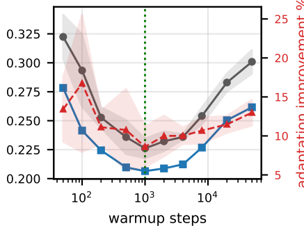
BDG2 / PatchTST
