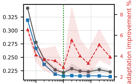
BDG2 / DLinear
