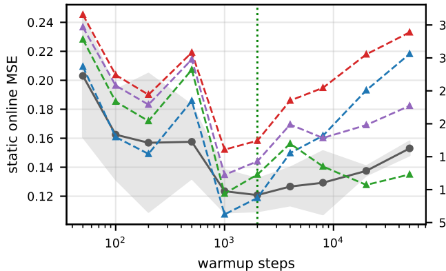
ETTm2 / PatchTST
