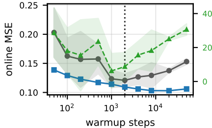
ETTm2 / PatchTST
