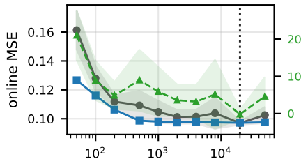
ETTm2 / PatchTST
