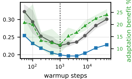
BDG2 / PatchTST
