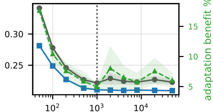
BDG2 / PatchTST
