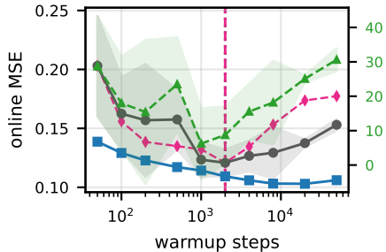
ETTm2 / PatchTST
