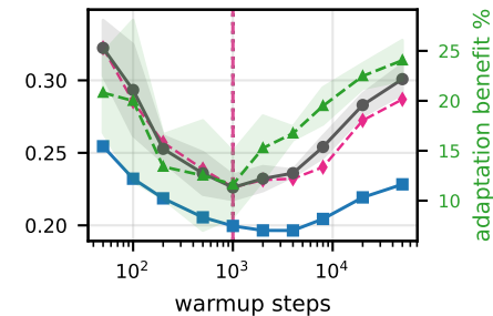
BDG2 / PatchTST
