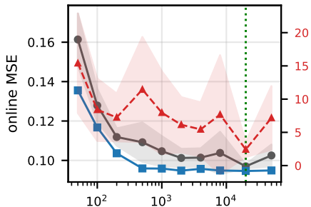
ETTm2 / PatchTST
