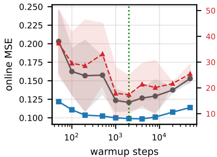
ETTm2 / PatchTST
