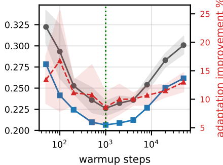
BDG2 / PatchTST
