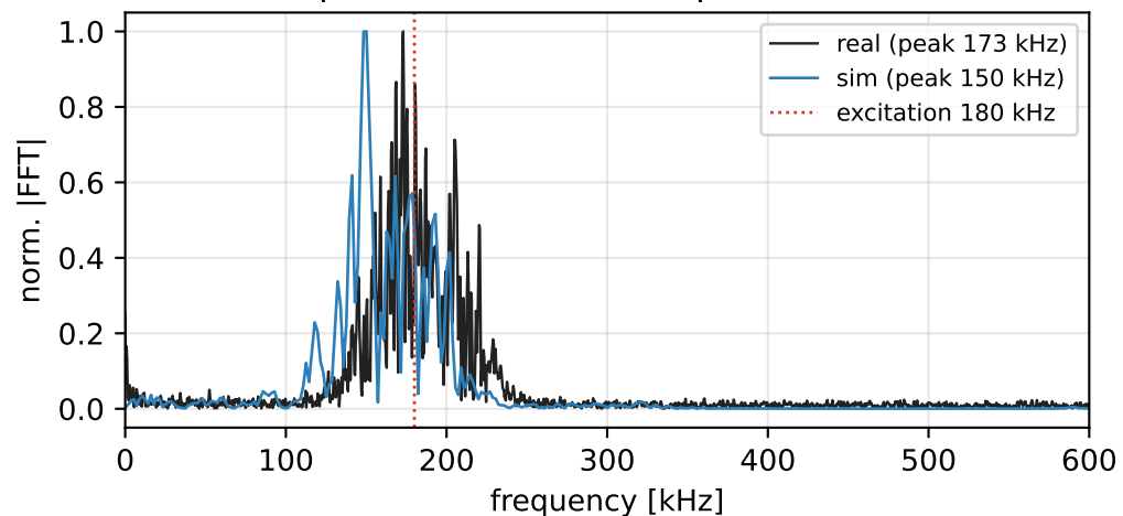
(d) spectra: dominant freq match [R vs S]
