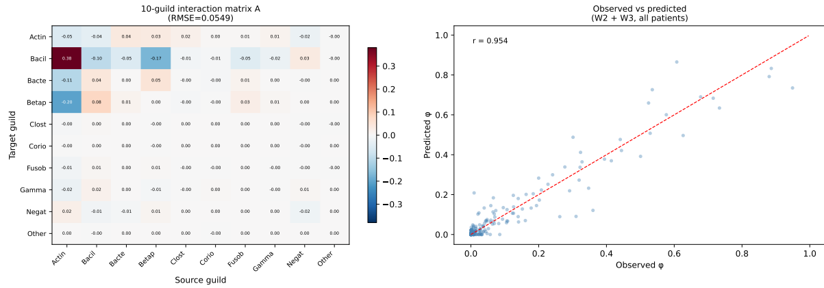
Figure 7: 左: 推定 10 \times 10 ギルド相互作用行列 (赤 = 正, 青 = 負). 右: 週 2 および 3 の観測値 vs. 予測値 ( r = 0.954 , RMSE = 0.055 ).
