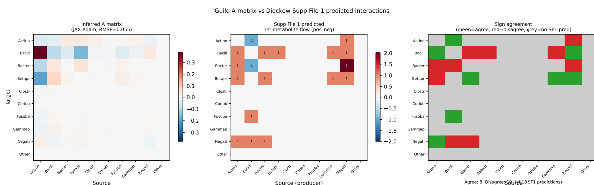
Figure 9: 推定ギルド A 行列と Dieckow Supp. File 1 予測相互作用の比較。左: 推定 A 行列 (JAX Adam, RMSE=0.055)。中: Supp. File 1 からの正味代謝フロースコア (正 = 正味 PRODUCES→USES; 負 = 正味 PRODUCES→IS_INHIBITED_BY)。右: 符号一致 (緑 = 一致, 赤 = 不一致, 灰 = Supp. File 1 予測なし)。18 予測ペアのうち 8 が一致, 10 が不一致。
