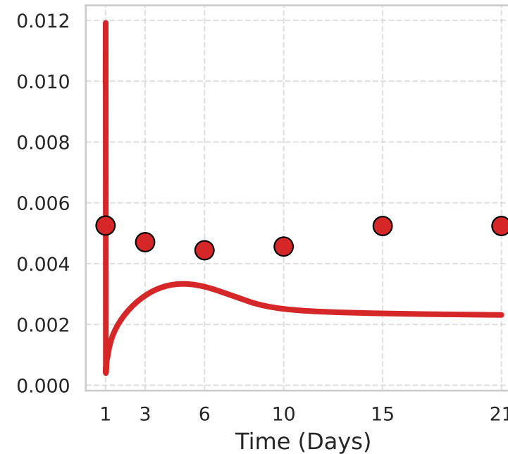
P. gingivalis
