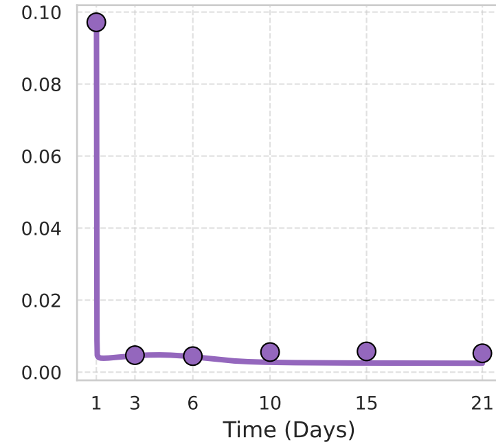
F. nucleatum
