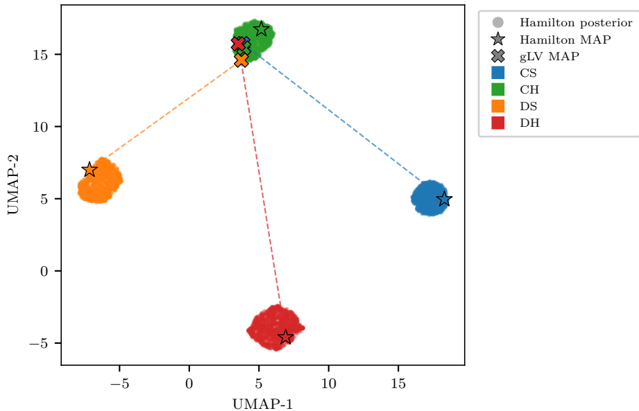
UMAP of A (Hamilton posterior + gLV MAP)
