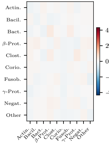
Langevin posterior mean
