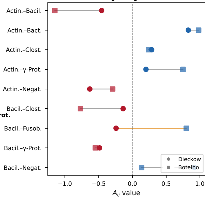
(B) Edge magnitudes
