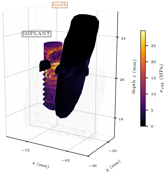
(B) occlusal von Mises \sigma_{vM}
