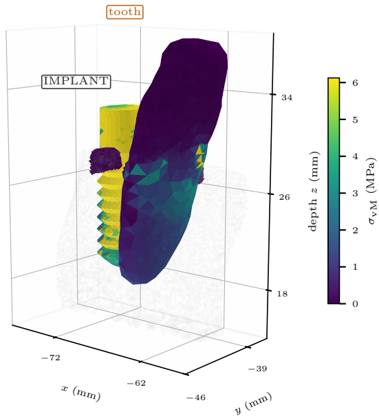
(B) occlusal von Mises \sigma_{vM}
