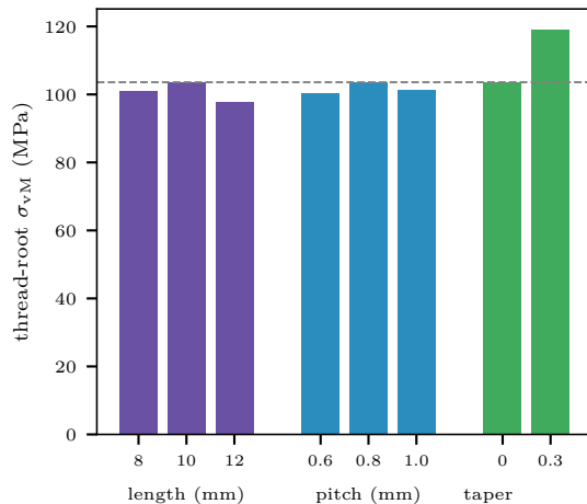
(D) C3D10 captures thread-root stress
