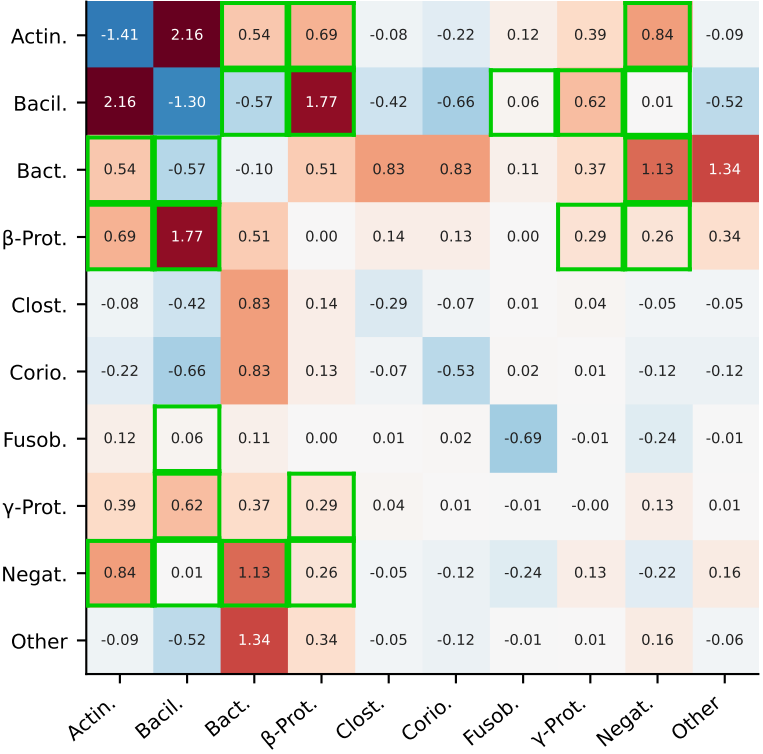
Hamilton + KEGG prior RMSE = 0.0830 r = 0.874 SA = 22/22
