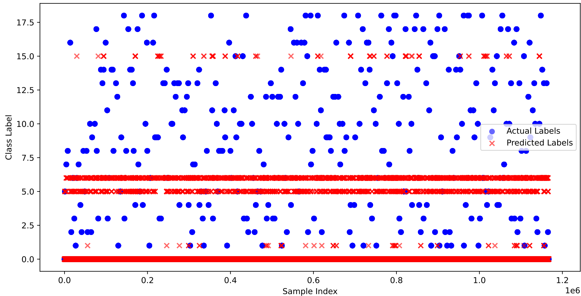
Predicted vs. Actual Class Labels
