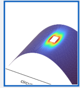
DSPSS field
