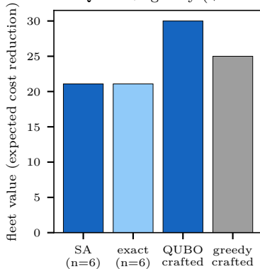
(b) SA = exact (gap 0.0) QUBO > greedy (+20)
