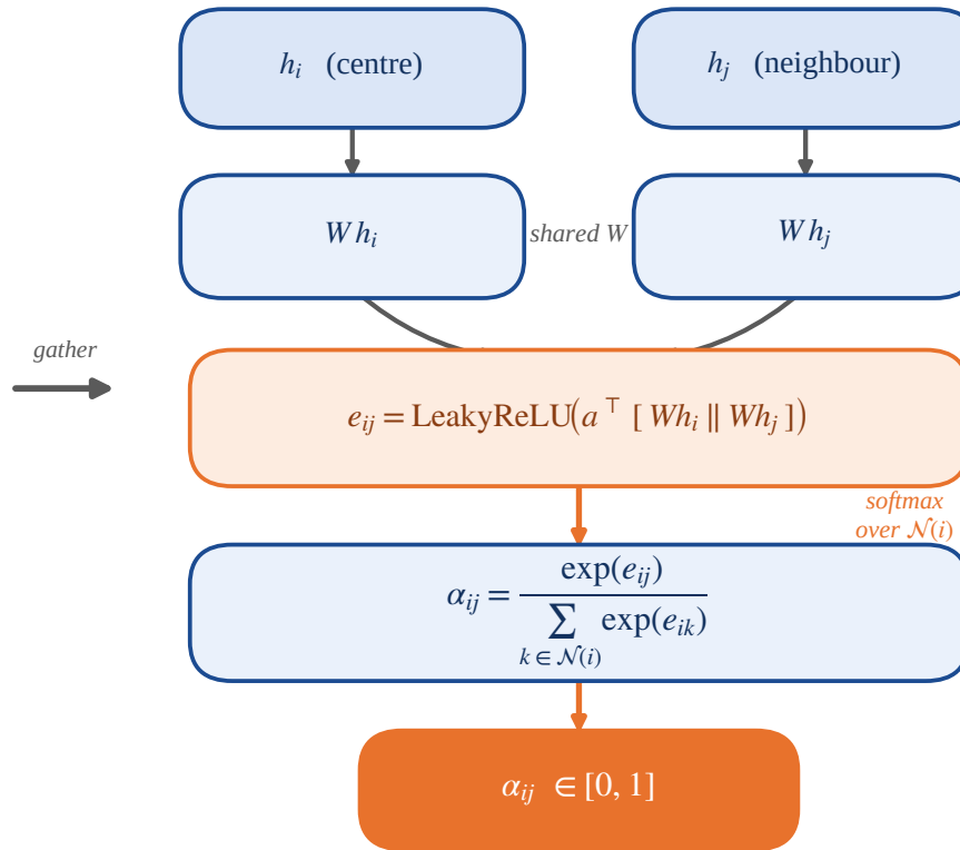
(B) Attention coefficient \alpha_{ij}
