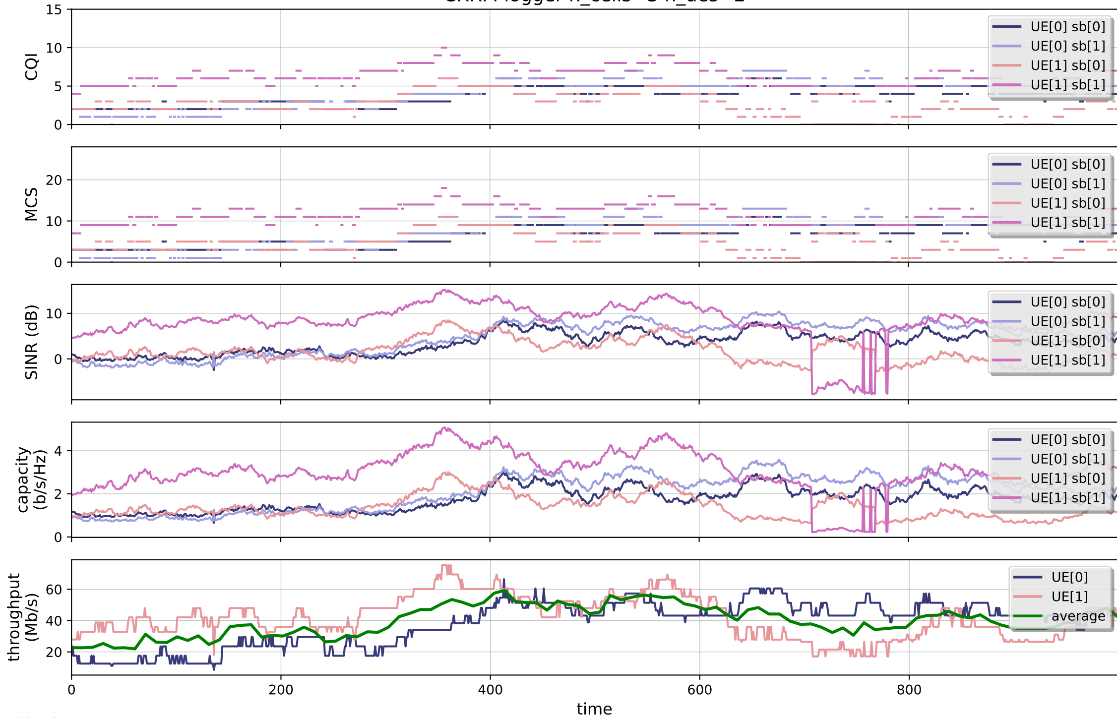
CRRM logger n_cells=3 n_ues=2
