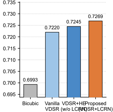
SSIM ↑
