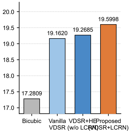
PSNR (dB) ↑
