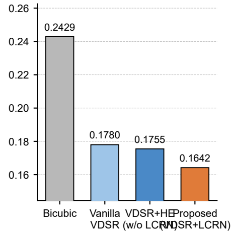
SAM (rad) ↓
