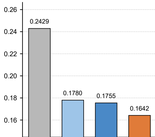
SAM (rad) ↓
