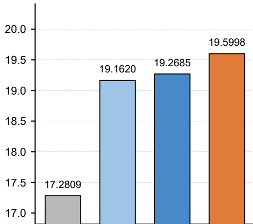
PSNR (dB) ↑
