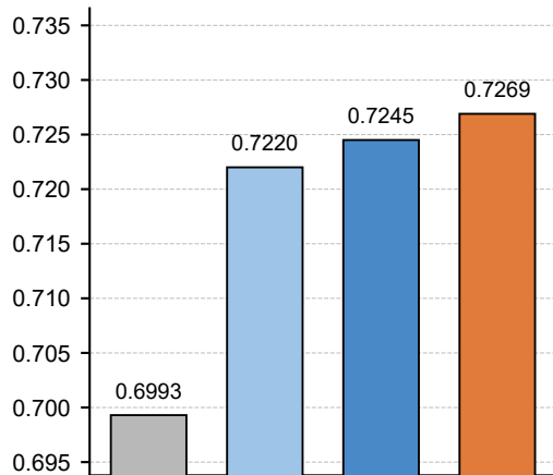
SSIM ↑
