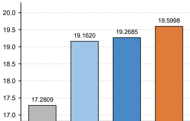
PSNR (dB) ↑
