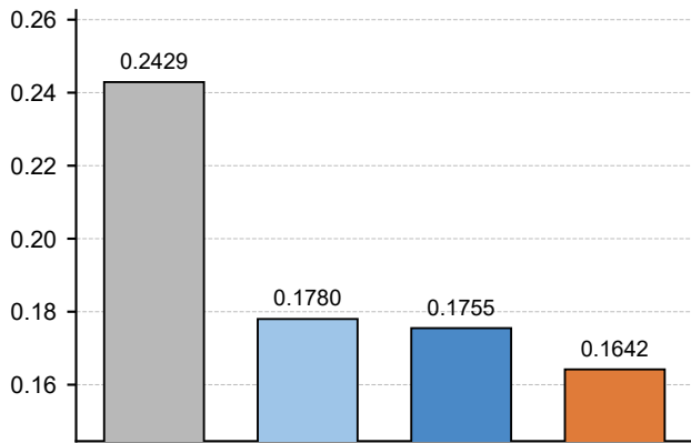
SAM (rad) ↓
