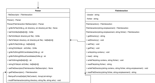
FIGURE 5 – Le diagramme UML représentant la classe Parser
