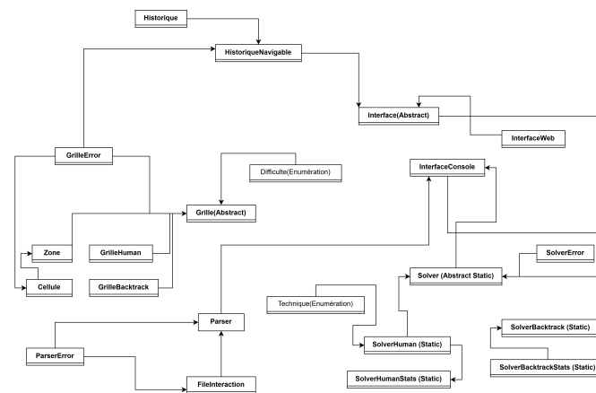
FIGURE 7 – Le diagramme UML entier et simplifié
