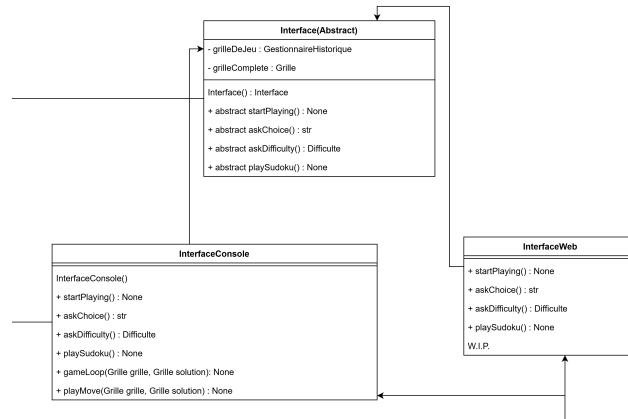
FIGURE 6 – Le diagramme UML représentant les classes d'Interface
