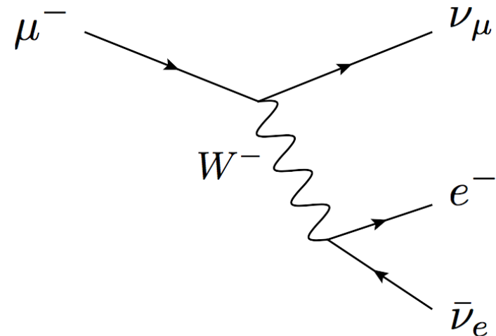
ミューオン崩壊のファインマン図
