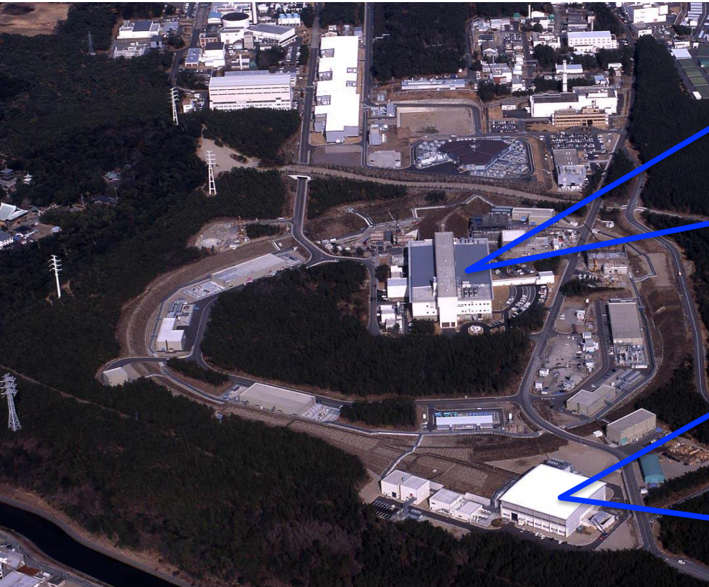
J-PARC @ 茨城県東海村
