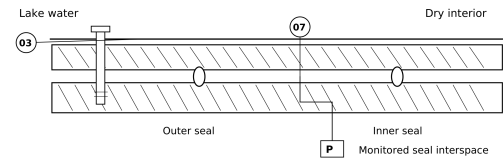
(d) Lid seal and shell detail
