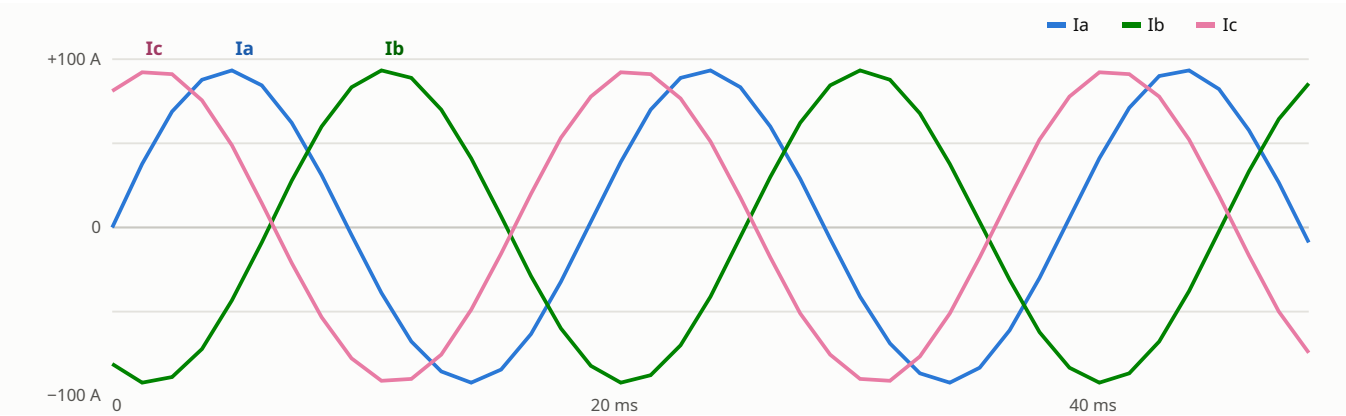
Fig. 5 — Visor SV: corrientes trifásicas 9-2LE (4000 muestras/s, 50 Hz) desfasadas 120°.
