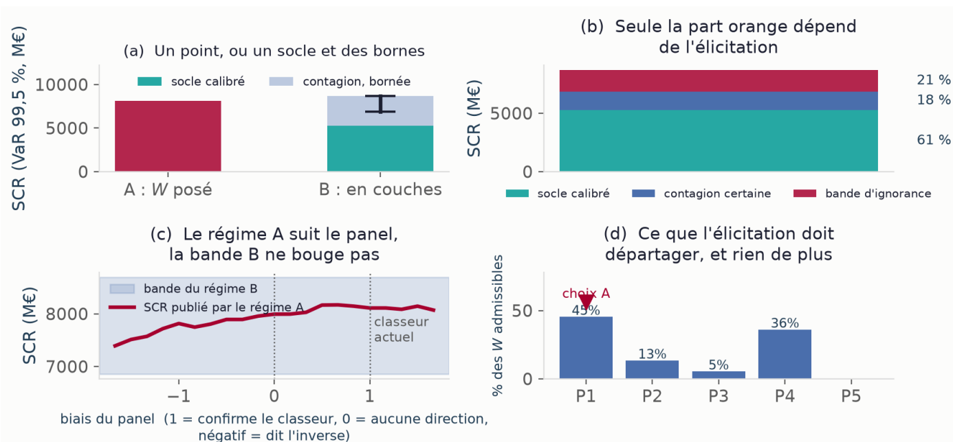
FIGURE J.9. Poser W ou le borner, comparés avant élicitation. (a) Un point contre un socle et des bornes. (b) Seule la part supérieure dépend de l'élicitation. (c) Le régime A suit le biais du panel, la bande du régime B ne bouge pas. (d) Ce que l'élicitation doit départager, et rien de plus.
