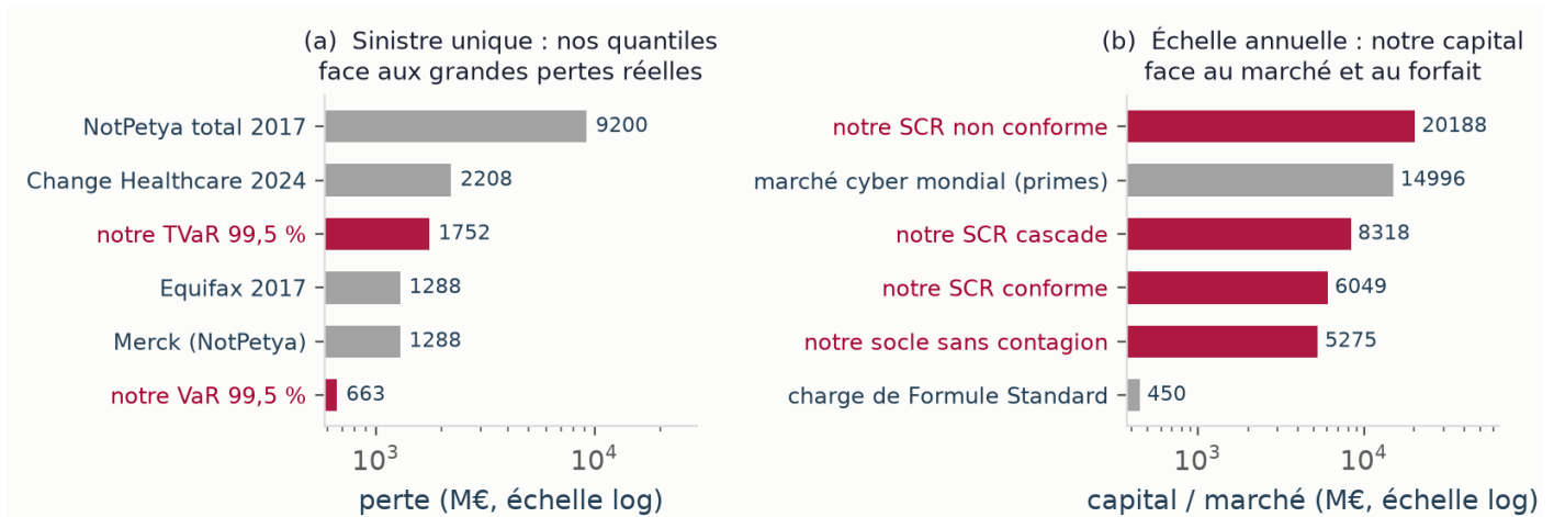
FIGURE J.12. Benchmark externe : la confrontation au réel, à deux échelles qu'il ne faut pas confondre. (a) au niveau du sinistre unique , les quantiles du modèle (quantile de sévérité 663 M€ et moyenne de queue 1 752 M€ à 99,5 %, et non des capitaux) s'insèrent parmi les grandes pertes cyber réelles, encadrant Merck-NotPetya, Equifax et Change Healthcare tout en restant sous le choc systémique NotPetya : la brique de sévérité est crédible. (b) à l'échelle annuelle , le capital est d'ordre systémique, comparable au marché cyber mondial, et domine de loin la charge de Formule Standard. C'est l'agrégation à une fréquence sectorielle, non la sévérité, qui porte l'agrégat à une échelle de secteur.
