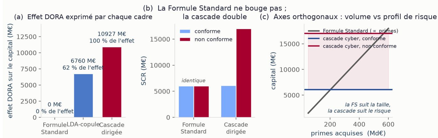
FIGURE J.10. Ce que chaque cadre exprime de l'effet DORA : 0 % pour la Formule Standard, 62 % pour la copule, 100 % pour la cascade.
