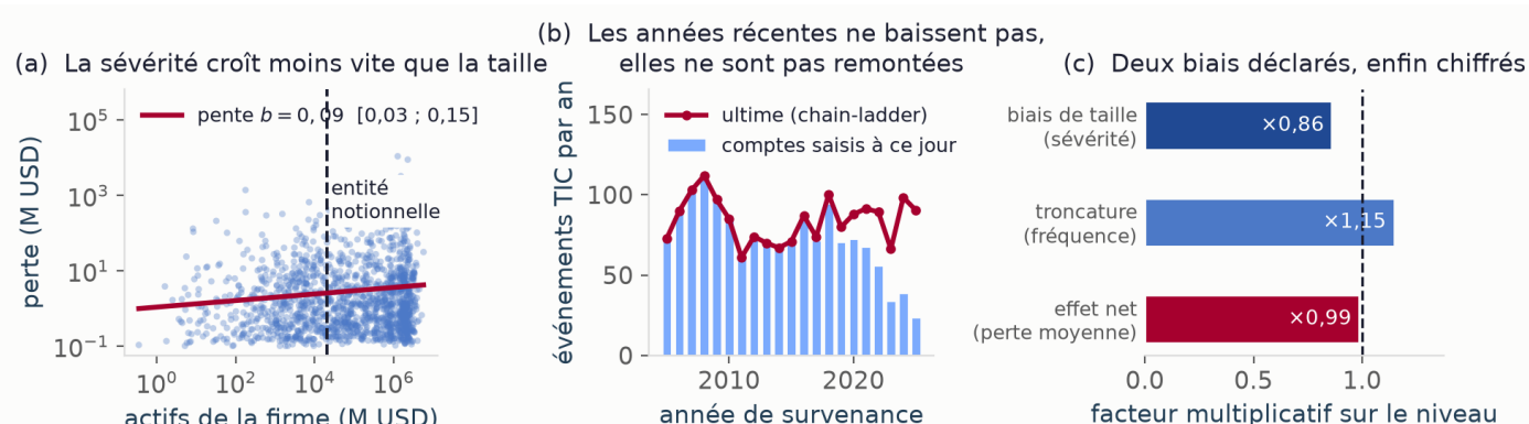
FIGURE J.4. Les deux biais, enfin chiffrés. (a) la sévérité croît beaucoup moins vite que la taille de la firme, et la pente brute est encore aplatie par le seuil de collecte. (b) les années récentes ne baissent pas, elles ne sont pas remontées : l'ultime chain-ladder les ramène au-dessus de la moyenne historique. (c) les deux corrections jouent en sens opposés.
