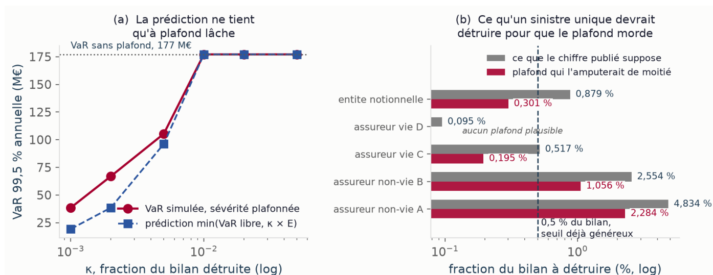
FIGURE I.7. Le plafond de sévérité adossé à l'exposition. (a) la prédiction naturelle, le quantile annuel borné par le plafond au titre du principe de la perte unique dominante, ne tient qu'à plafond lâche : plafonner détruit la queue lourde que ce principe suppose, et la charge redevient un cumul. (b) la première série donne la fraction du bilan qu'un sinistre unique devrait détruire pour que le besoin publié soit atteignable, la seconde le plafond qui ampute ce besoin de moitié. L'écart entre les deux barres est ce qui met la plus petite entité hors domaine, et l'entité la plus grande n'est amputée par aucun plafond discutable.
