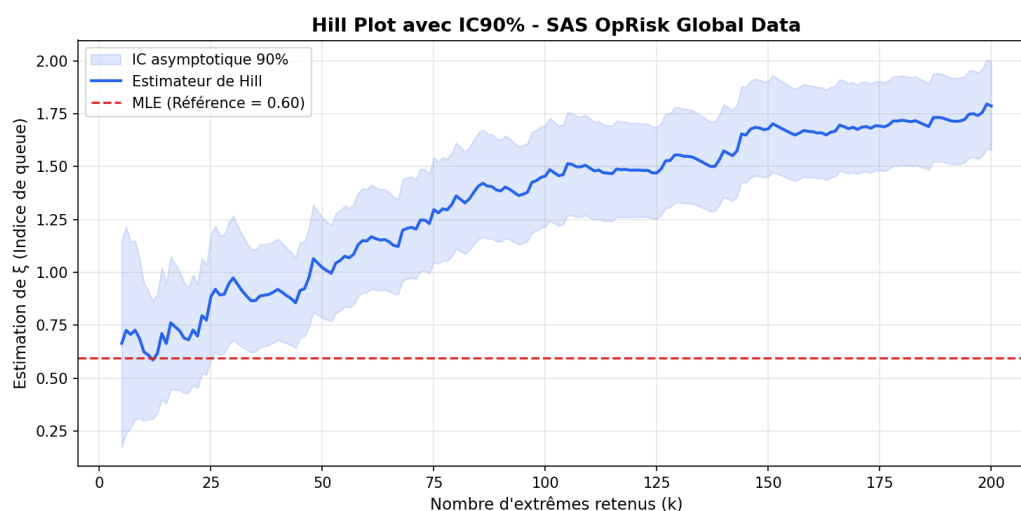
FIGURE J.5. Hill plot avec intervalle de confiance asymptotique à 90 % sur OpRisk Global. La référence MLE ( \hat{\xi} \approx 0,595 , pointillés rouges) n'est statistiquement compatible avec l'estimateur de Hill que pour k \leq 25 ; au-delà, la dérive de \hat{\xi}_{\text{Hill}} traduit le biais croissant lié à l'intégration d'observations hors du régime asymptotique pur de la queue.
