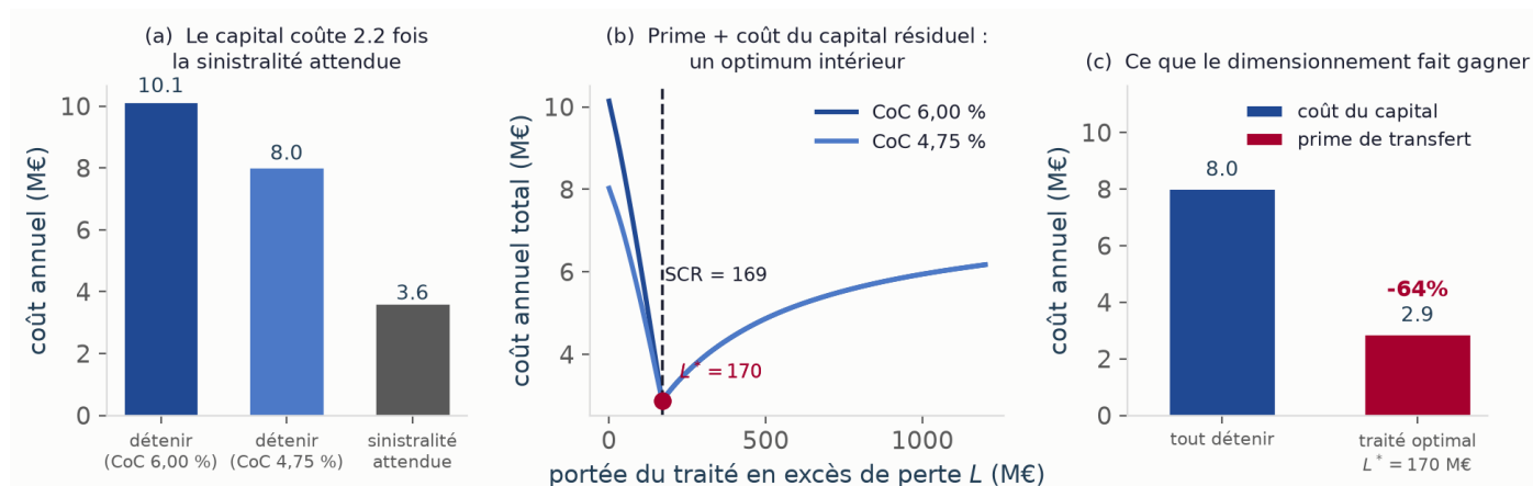
FIGURE J.13. Détenir ou transférer : le SCR confronté au prix de marché du même risque, à l'échelle d'entité corrigée. (a) le coût annuel du capital (8,0 M€ au taux révisé de 4,75 %) vaut 2,2 fois la sinistralité attendue (3,6 M€) : c'est ce rapport, absent de toute comparaison de niveau, qui rend le transfert pertinent. (b) le coût total, prime plus coût du capital résiduel, en fonction de la portée L du traité en excès de perte ; l'optimum tombe en L^* = \text{SCR} = 169 M€, là où le capital résiduel s'annule. (c) ce que le dimensionnement fait gagner, -64\% , chiffre à lire comme une borne supérieure : capacité de marché, exclusions et risque de contrepartie l'entament, mais il faudrait 78\% d'inefficacité pour renverser la conclusion.
