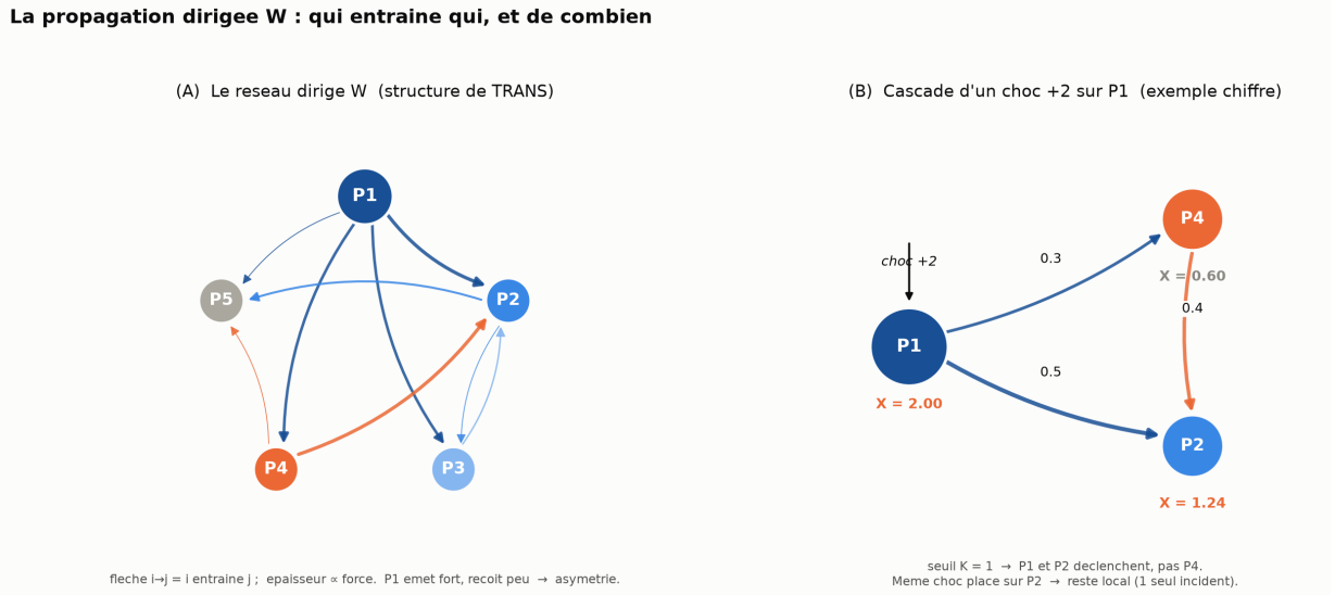
Figure 1. (A) La structure dirigée de W sur les 5 piliers : P1 émet fort et reçoit peu. (B) Le sous-réseau de l'exemple ci-dessous et la propagation d'un choc.
