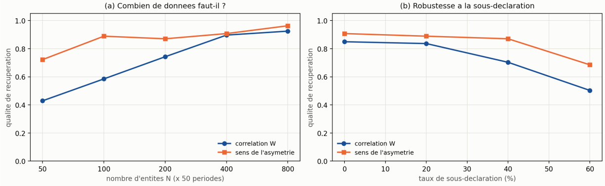
Figure 6. (a) Avec la contagion admissible (normalisée), quelques centaines d'entités ne suffisent plus : la corrélation passe de 0,43 ( N = 50 ) à 0,90 ( N = 400 ), et le sens de l'asymétrie de 72 % à 91 % des paires. (b) La récupération se dégrade progressivement avec la sous-déclaration (corrélation 0,85 \rightarrow 0,50 entre 0 % et 60 %), et le sens de la propagation se dégrade aussi (91 % \rightarrow 69 %).
