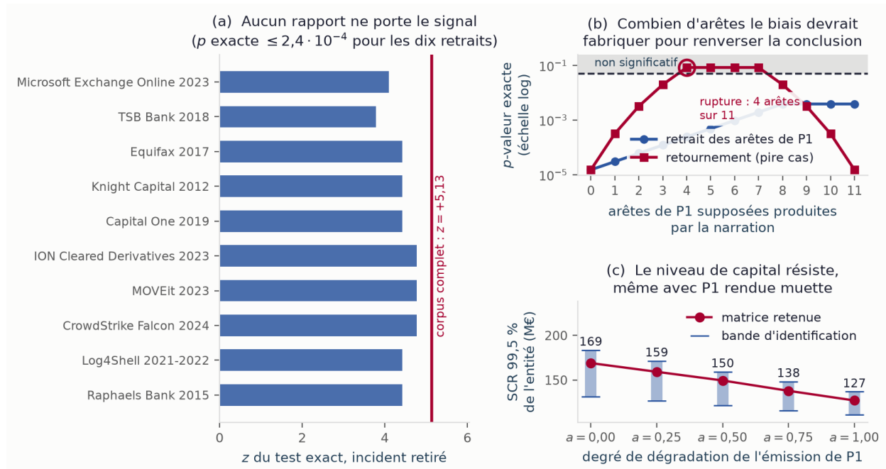
FIGURE I.10. Le biais de narration, mesuré au lieu d'être déclaré. (a) jackknife par incident : aucun rapport ne porte le signal à lui seul, les dix retraits laissant p \leq 2,4 \cdot 10^{-4} . (b) point de rupture, en p -valeur exacte et non en z : il faudrait quatre arêtes de P_1 retournées dans la pire configuration pour perdre la significativité, et aucun nombre de retraits n'y suffit. La courbe de retournement remonte au-delà de sept parce que retourner toutes les arêtes n'efface pas l'asymétrie, elle l'inverse. (c) le niveau de capital résiste, y compris avec P_1 rendue muette, et la bande d'identification se resserre à mesure que l'émission de P_1 disparaît.
