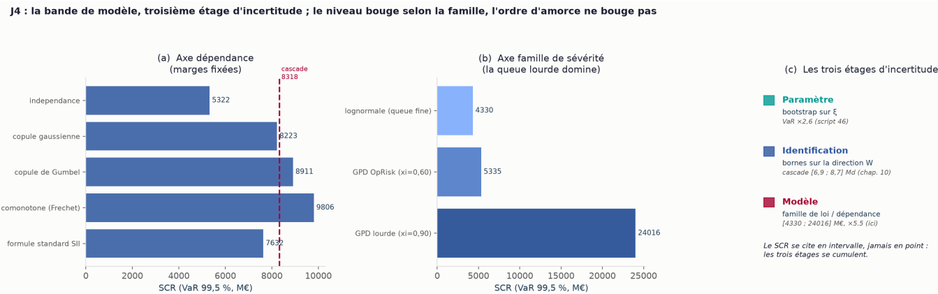
Figure 11.1. La bande de modèle, troisième étage d'incertitude. (a) axe dépendance, à marges fixées : la cascade se place entre les copules gaussienne et de Gumbel, dans une bande [5,3 ; 9,8] Md€. (b) axe famille de queue : la queue lourde domine l'incertitude ( \times 5,5 ). (c) les trois étages (paramètre, identification, modèle) tels que le script les cumule ; la bande reportée par le mémoire n'en retient que les deux premiers, le troisième étant publié comme axe de sensibilité (§11.2.1). Source : script 48.
