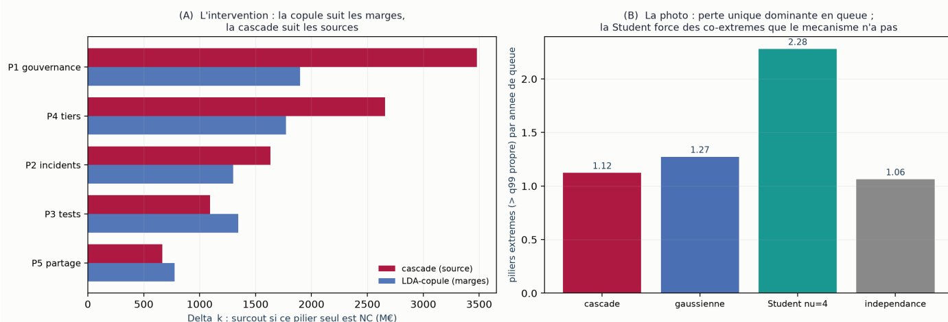
Figure 10.7. Benchmark copule (OpRisk). (A) Intervention : le jeu copule suit les marges et sous-estime le surcoût, la cascade suit les sources. (B) Photo : perte unique dominante en queue ; la Student force des co-extrêmes que le mécanisme n'a pas. Source : script 23.
