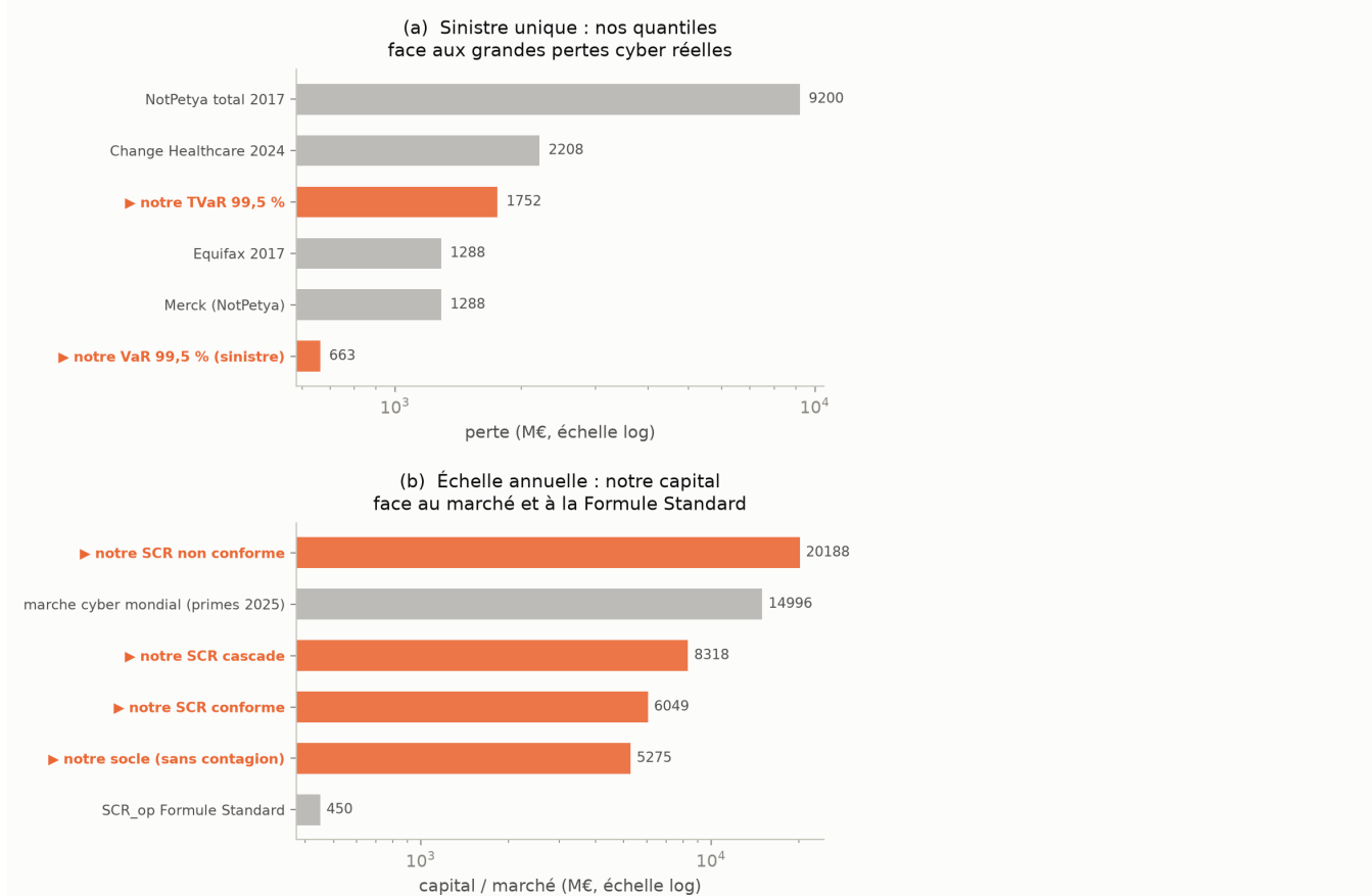
Figure 10.10. Benchmark externe : la confrontation au réel, à deux échelles qu'il ne faut pas confondre. (a) au niveau du sinistre unique , nos quantiles (VaR 663 M€ et TVaR 1 752 M€ à 99,5 %) s'insèrent parmi les grandes pertes cyber réelles, encadrant Merck-NotPetya, Equifax et Change Healthcare tout en restant sous le choc systémique NotPetya : la brique de sévérité est crédible. (b) à l'échelle annuelle , le capital est d'ordre systémique, comparable au marché cyber mondial, et domine de loin la charge de Formule Standard. C'est l'agrégation à une fréquence sectorielle, non la sévérité, qui porte l'agrégat à une échelle de secteur. Source : script 49.
