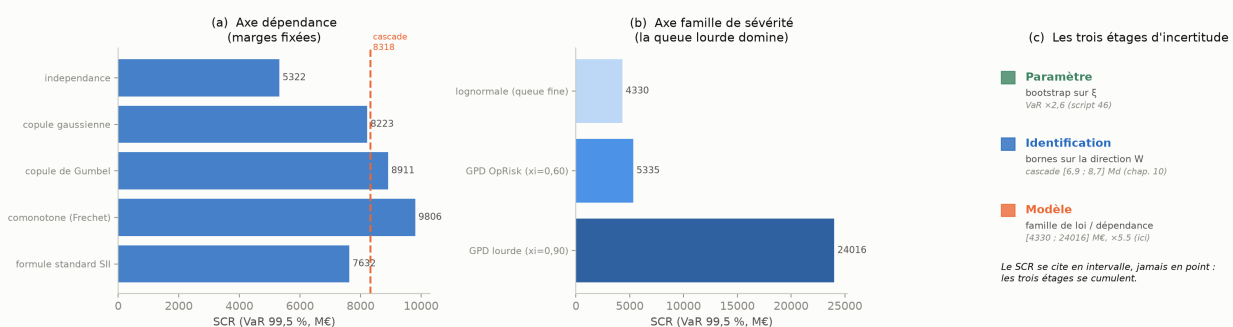
Figure 1. (a) axe dépendance, à marges fixées : la cascade se place entre les copules gaussienne et de Gumbel. (b) axe famille de queue : la queue lourde domine l'incertitude. (c) les trois étages (paramètre, identification, modèle) se cumulent.
