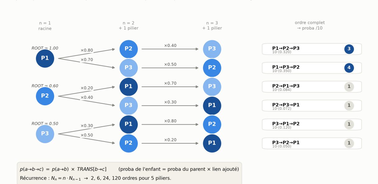
Figure 1. La probabilité se construit lien par lien le long de l'arbre des ordres : proba de l'enfant = proba du parent \times transition ajoutée. L'asymétrie de TRANS (p.ex. P1→P3 à 0,70 contre P3→P1 à 0,30) est ce qui sépare les verdicts. N.B. seule la probabilité se décompose ainsi ; la gravité, elle, dépend de l'ensemble des piliers présents (étendue) et n'est pas multiplicative le long de l'arbre.
