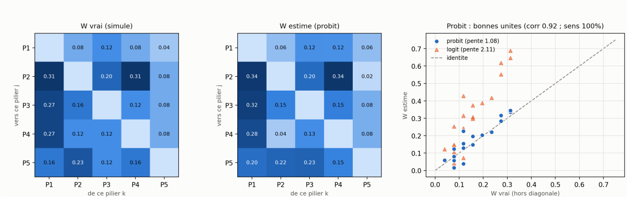
Figure 5. Sur un panel simulé (800 entités \times 60 périodes), le probit retrouve W dans ses propres unités : corrélation 0,92, pente 1,08, sens de l'asymétrie correct pour 100 % des paires. Le logit, lui, gonfle systématiquement les coefficients.
