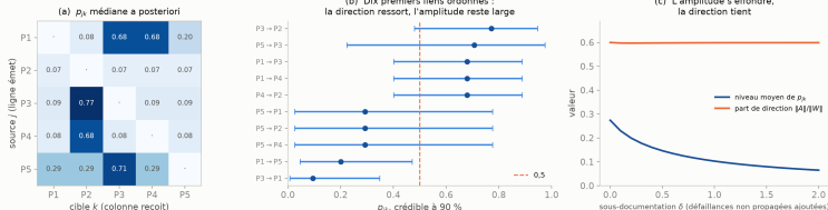
Z20 : corpus étendu à 10 post-mortems, et matrice ordonnée p_{jk} au lieu du seul sens par paire
