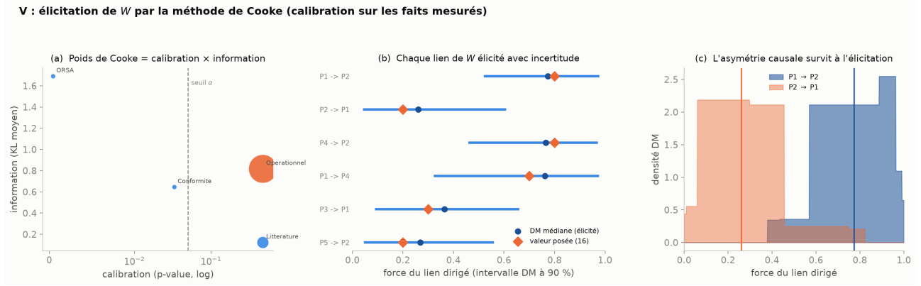
Figure 1. Démonstration sur experts fictifs de profils contrastés. (a) L'expert bien calibré et informatif domine ; le sur-confiant et le biaisé passent sous le seuil \alpha . (b) Chaque lien de W ressort avec un intervalle à 90 % autour de la valeur posée. (c) L'asymétrie causale P1 \rightarrow P2 vs P2 \rightarrow P1 survit à l'élicitation.
