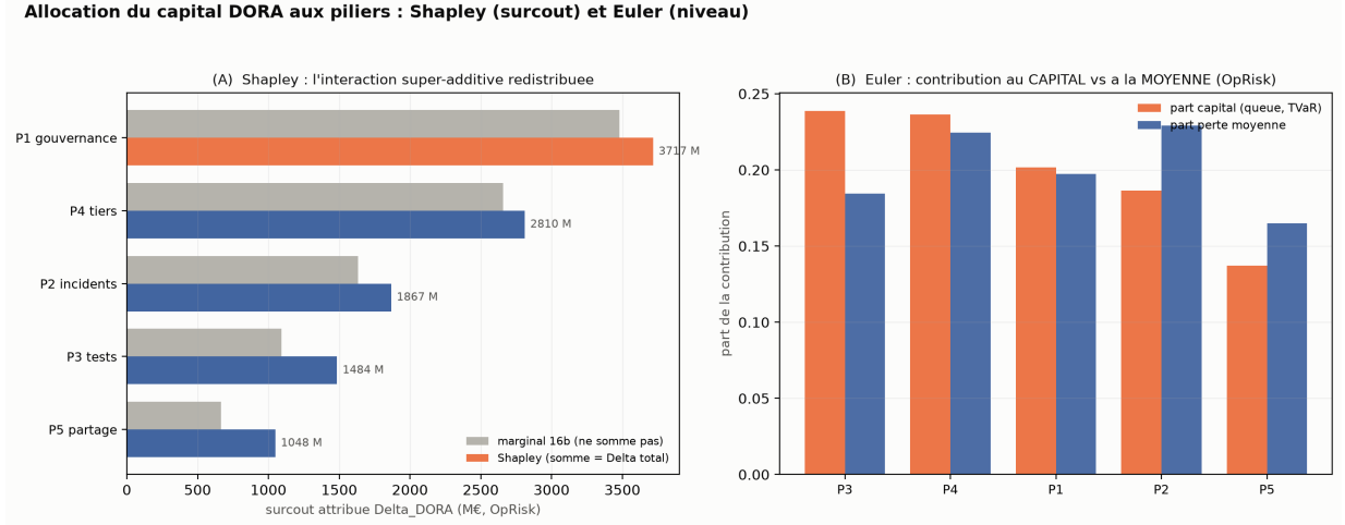
Figure 8.3. Allocation du capital DORA (OpRisk). (A) Shapley contre marginaux : l'interaction redistribuée. (B) Euler : parts de capital (queue) contre parts de perte moyenne ; sur ce périmètre non plafonné, l'allocation fine de la queue extrême reste indicative ( \xi \approx 0,6 , variance de sévérité infinie). Source : script 20.
