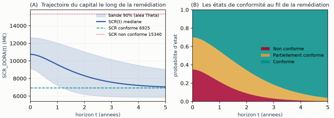
Figure 10.4. Trajectoire \text{SCR}(t) et évolution des états de conformité.
