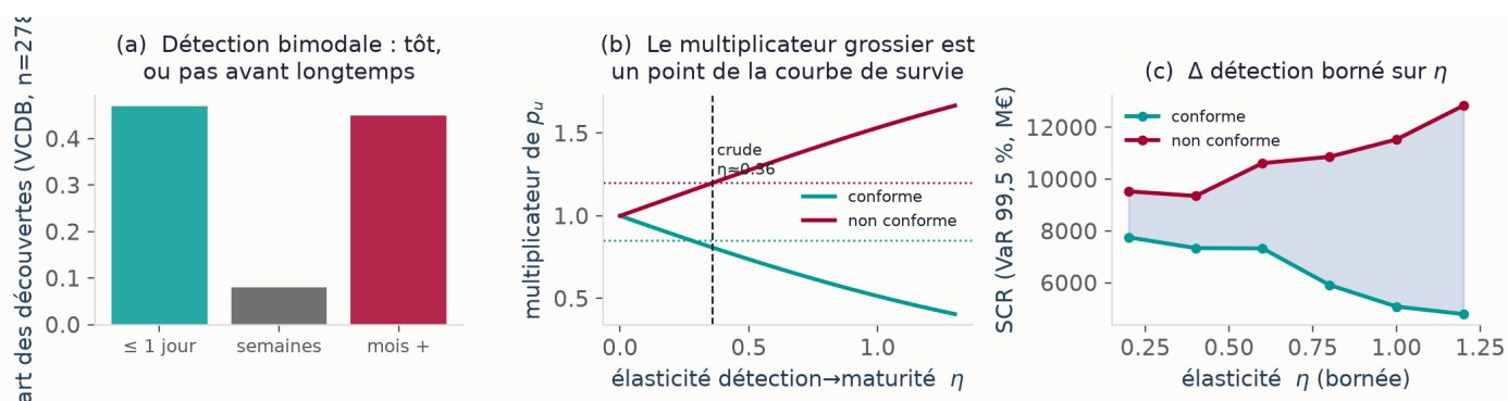
Figure B.6. P2/P3, la détection comme courbe de survie. (a) La distribution bimodale observée au VCDB. (b) Le multiplicateur de matérialité comme point de la courbe de survie ; le multiplicateur grossier actuel correspond à \eta \approx 0,36 . (c) Le surcoût du canal détection, borné sur l'élasticité.
