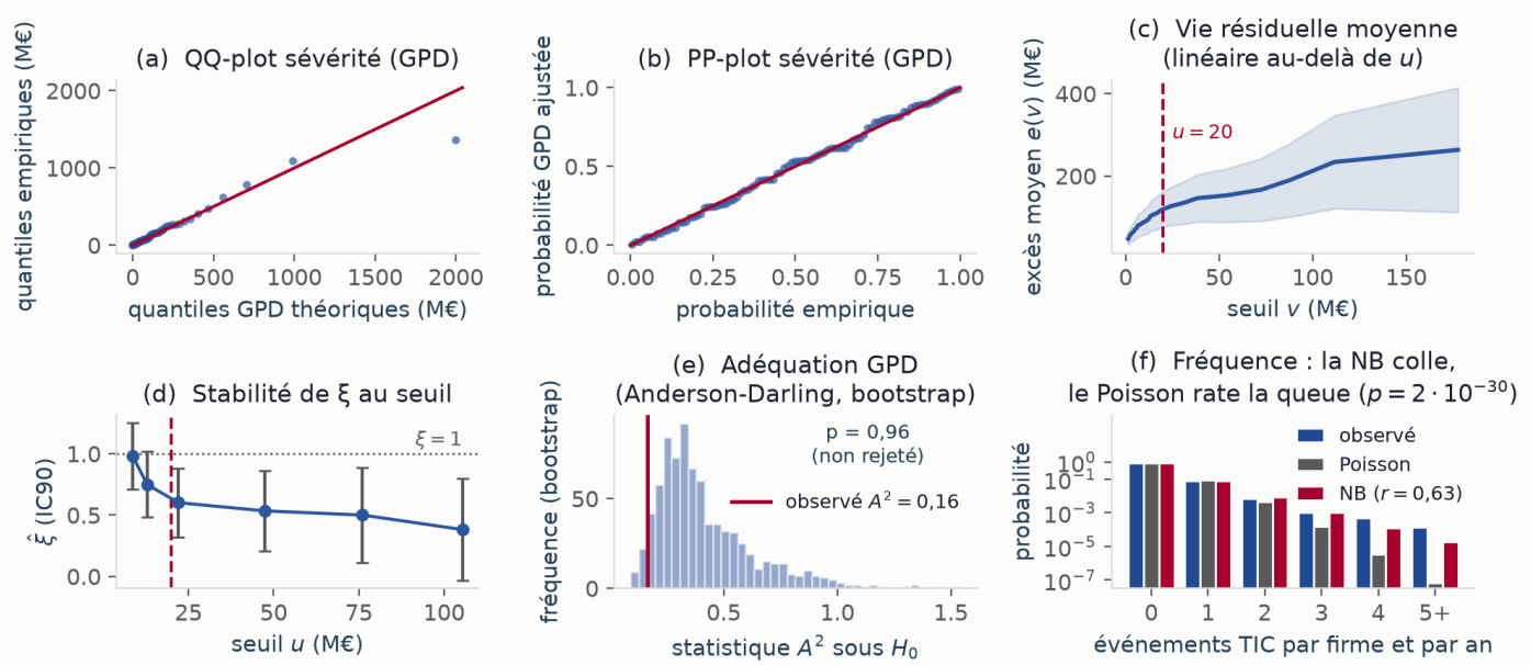
Figure 5.3. Validation du socle. (a-b) QQ-plot et PP-plot de la sévérité contre la GPD ajustée. (c) vie résiduelle moyenne, linéaire au-delà de u . (d) stabilité de \hat{\xi} au seuil. (e) test d'Anderson-Darling, loi nulle par bootstrap paramétrique et statistique observée ( p = 0,96 ). (f) adéquation de la fréquence : la NB colle aux comptes firme-année, le Poisson rate la queue ( p = 2 \cdot 10^{-30} ).
