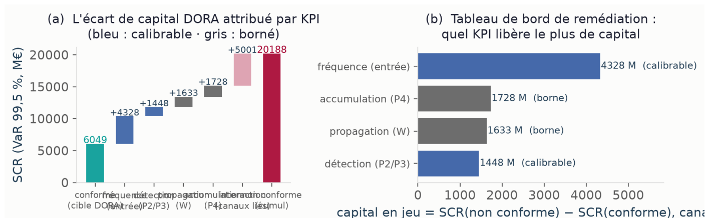
Figure B.8. Des KPI descriptifs aux KPI pilotables. (a) l'écart de capital DORA attribué par KPI, chaque canal isolé (bleu : calibrable ; gris : borné), avec l'interaction qui referme la cascade. (b) le tableau de bord de remédiation, les KPI classés par capital libéré.
