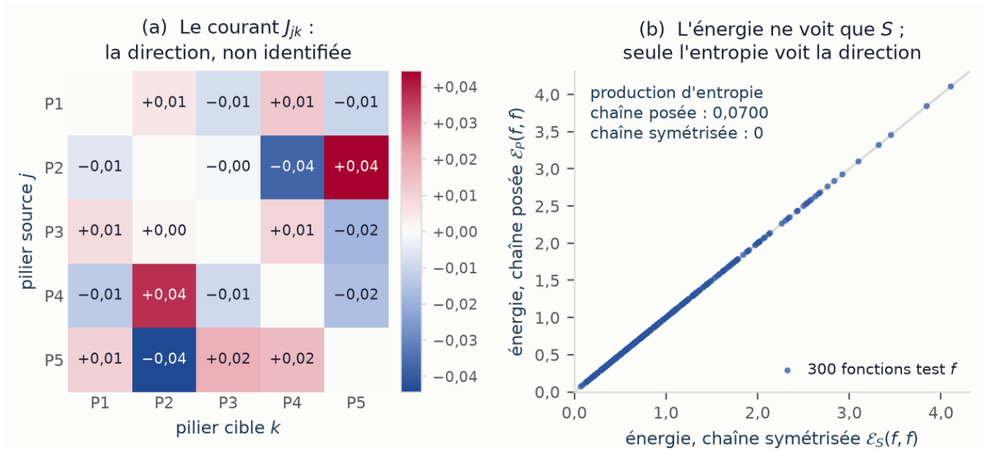
Figure 8.1. La direction A comme courant irréversible, et pourquoi une statistique invariante par renversement ne peut pas la voir. (a) le courant J_{jk} = \pi_j P_{jk} - \pi_k P_{kj} est non nul : le modèle porte bien une direction. (b) pour trois cents fonctions test tirées au hasard, l'énergie de fluctuation, c'est-à-dire la variation quadratique de la martingale, est la même pour la chaîne posée et pour sa symétrisée : les points tombent sur la diagonale, elle ne voit que S . Seule la production d'entropie distingue les deux chaînes, et elle s'annule à la symétrisation.
