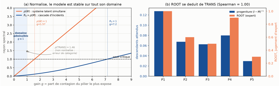
Figure 6.2. (a) Sur le domaine admissible g \leq 1 , les deux rayons spectraux restent < 1 ; les seuils critiques ( \rho(W) = 1 à g = 1,57 ; R_0 = 1 à g = 7,2 ) sont hors domaine. (b) La progéniture (I - M)^{-1} reproduit exactement le classement ROOT du jugement d'expert. Source : 03_calibration_W.
